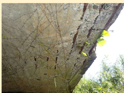
▲RC橋（鉄筋露出）
